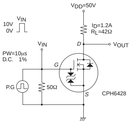
スイッチングタイム測定回路図
