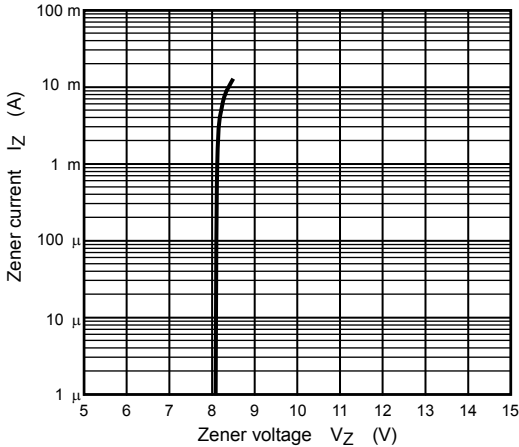
I_Z - V_Z
