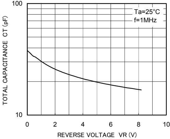
CT - V_R
