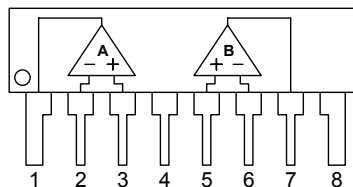
NJM12904L
