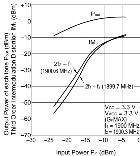
OUTPUT POWER AND IM 3 vs. INPUT POWER
