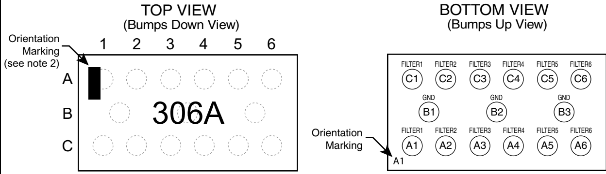
CSPEMI306A CSP Package
