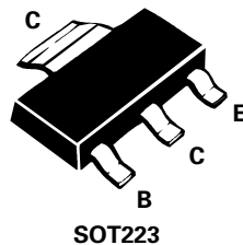
SOT223
