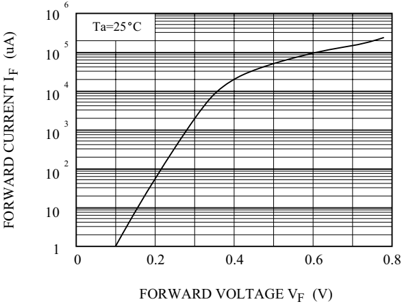
I_F - V_F
