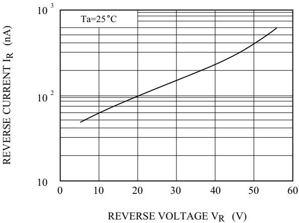
I_R - V_R
