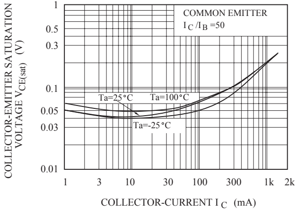
V_{CE(sat)} - I_C
