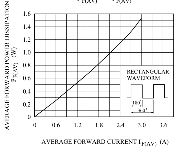
P_{F(AV)} - I_{F(AV)}
