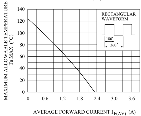
T_a - I_{F(AV)}
