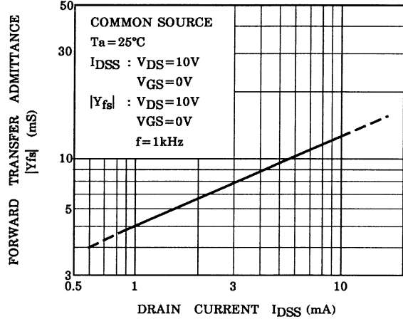
|Y_{fs}| - I_{DSS}
