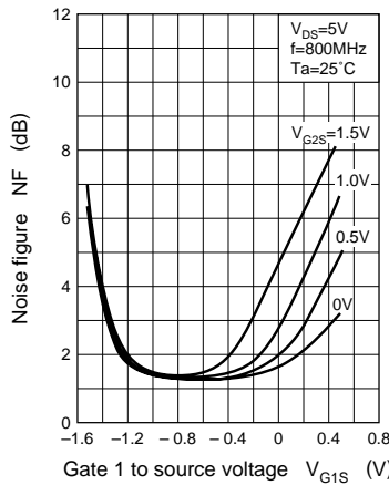
NF - V_{G1S}
