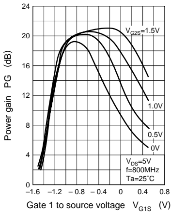
PG - V_{G1S}
