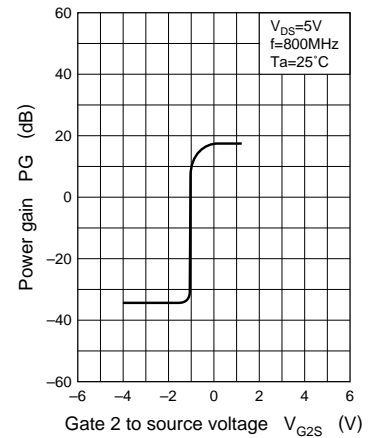
PG - V_{G2S}
