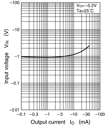
V_{IN} - I_O
