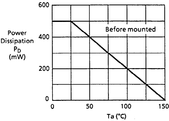
(2) SOT-89-3
