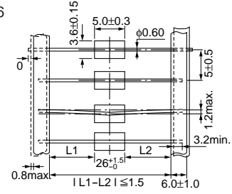
BL01RN1-A63T6
