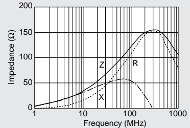
BLM31P121SG
